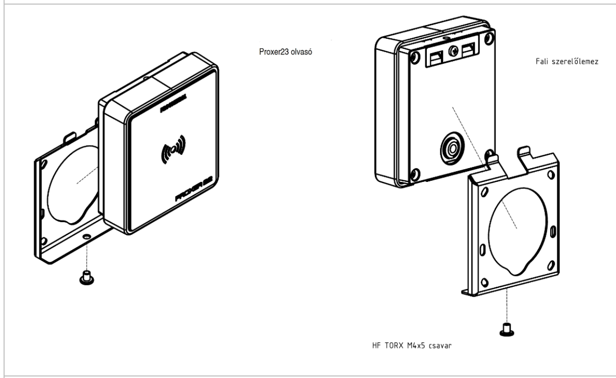
1781-16-21 fali szerelőlemez
